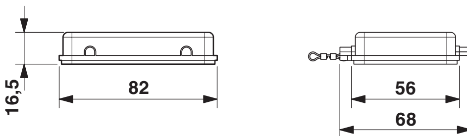
Disegno quotato
