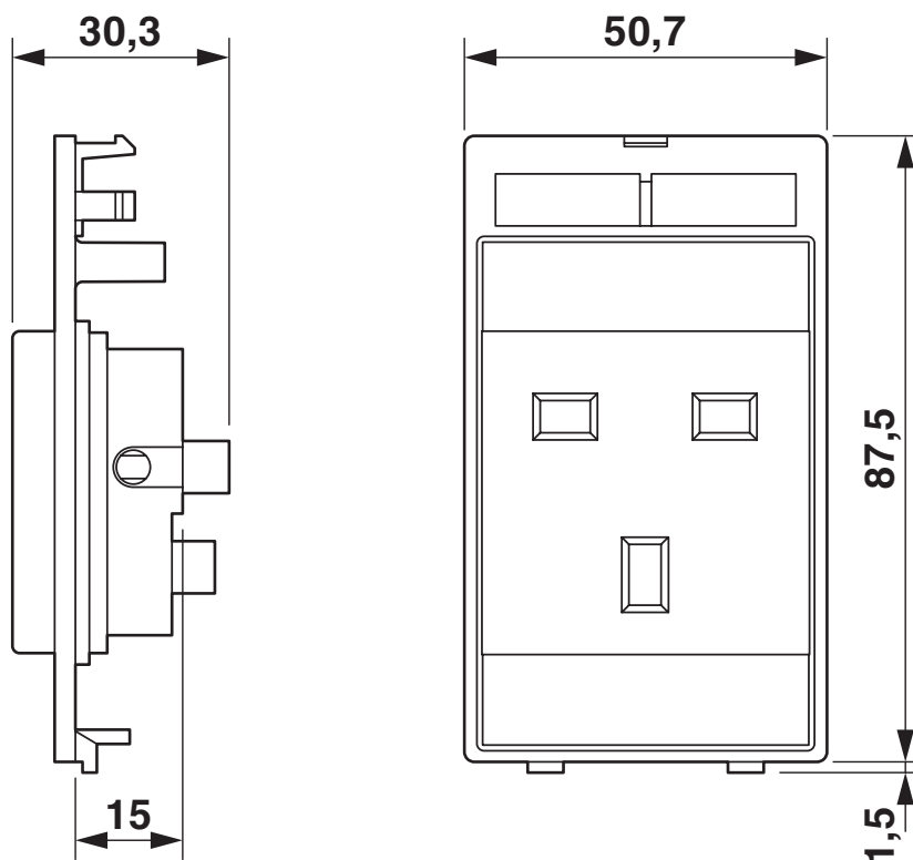
Disegno quotato
