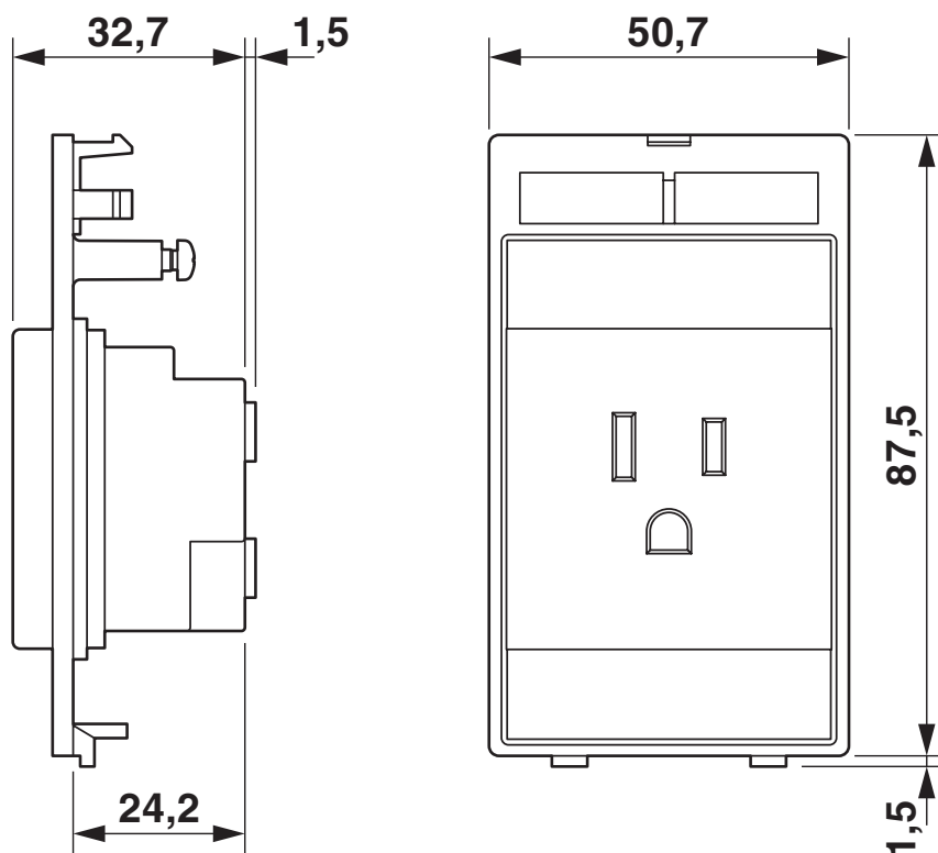
Disegno quotato
