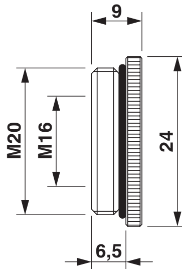
Disegno quotato
