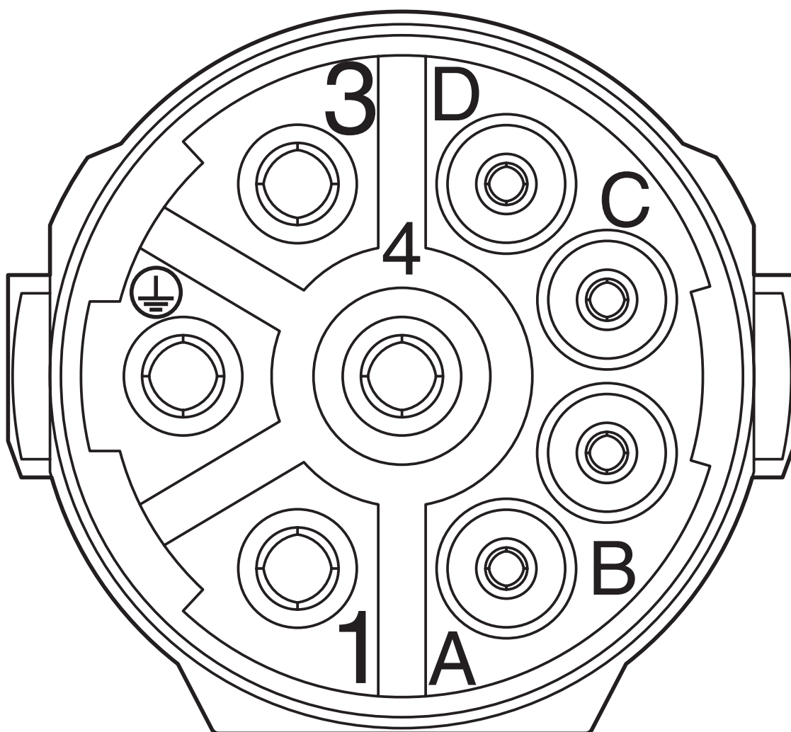
Disegno schema
