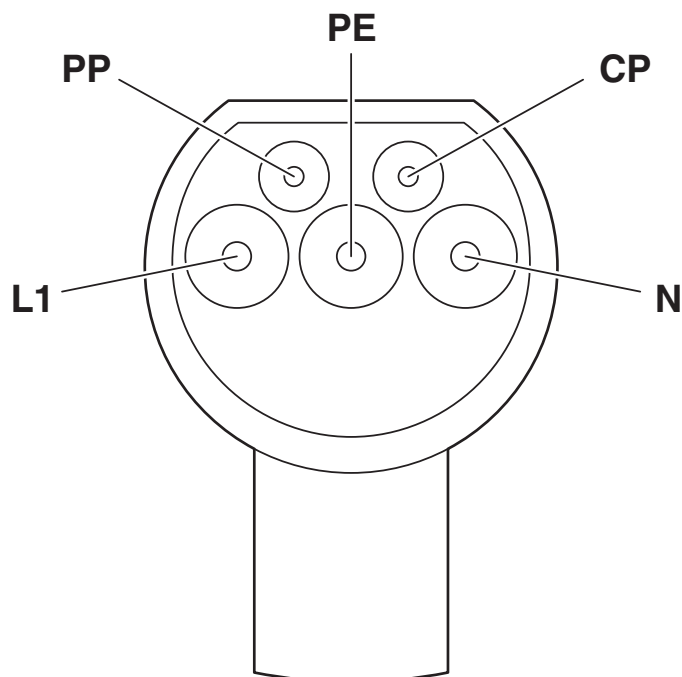
Disegno collegamento
