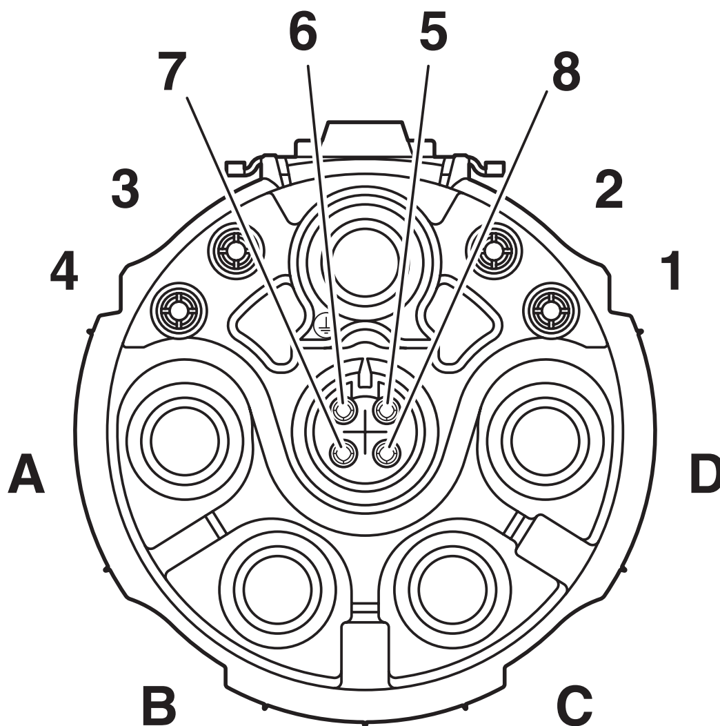
Disegno schema
