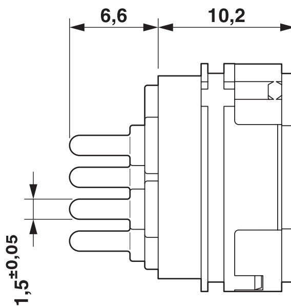
Disegno quotato
