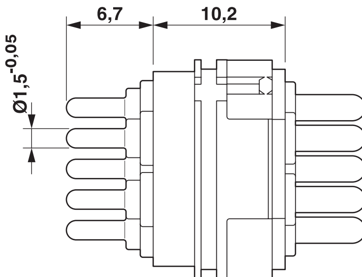
Disegno quotato
