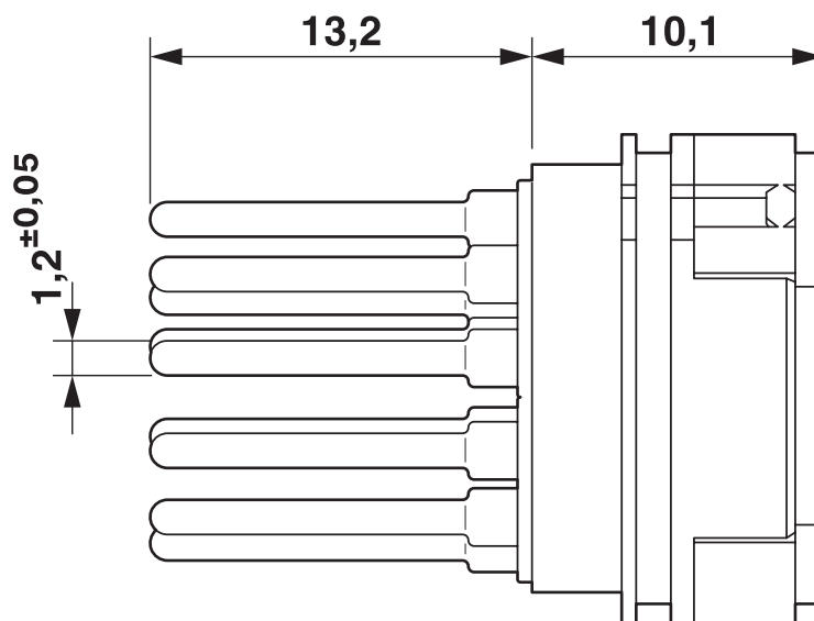
Disegno quotato
