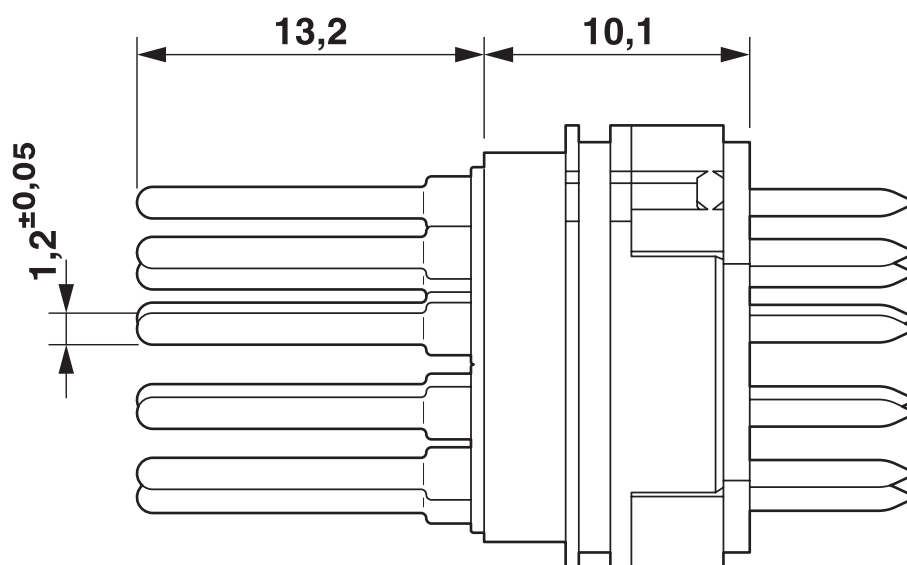
Disegno quotato
