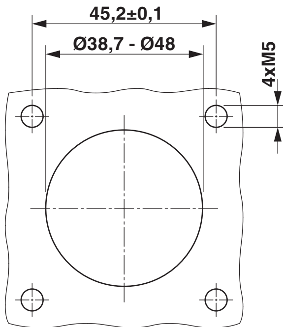
Dima di forat./geometria di pad di saldat.
