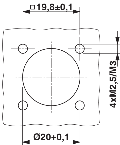
Disegno quotato
