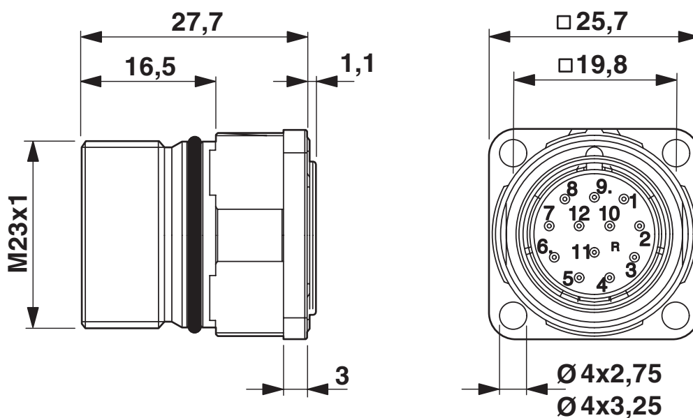
Disegno quotato
