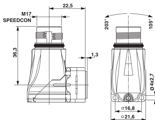
Disegno quotato
