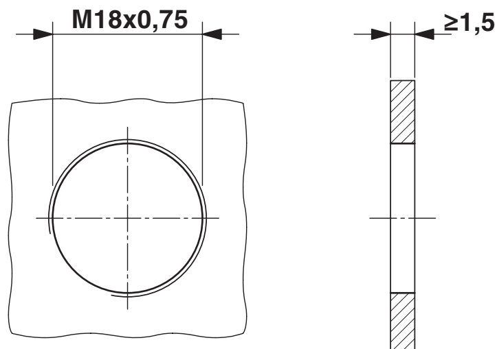
Disegno quotato
