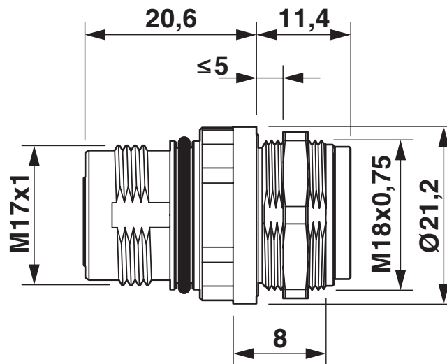
Disegno quotato
