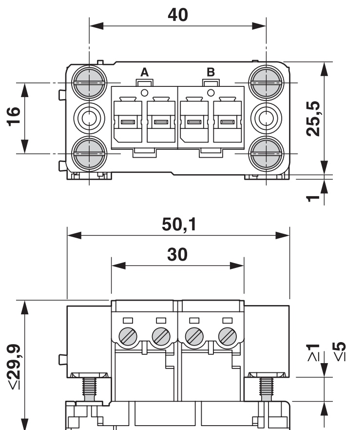
Disegno quotato
