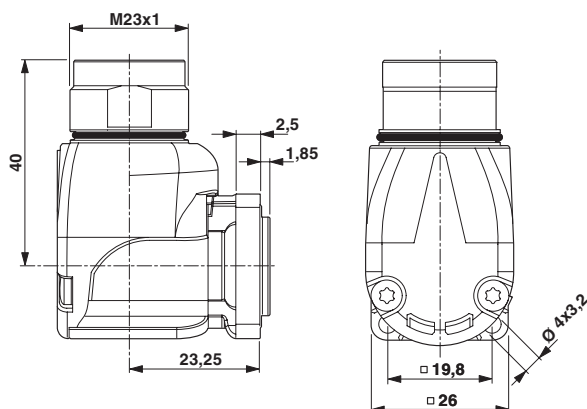
Disegno quotato
