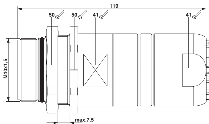
Disegno quotato
