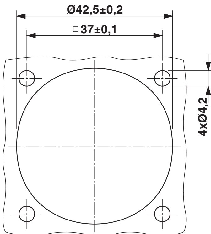
Disegno quotato
