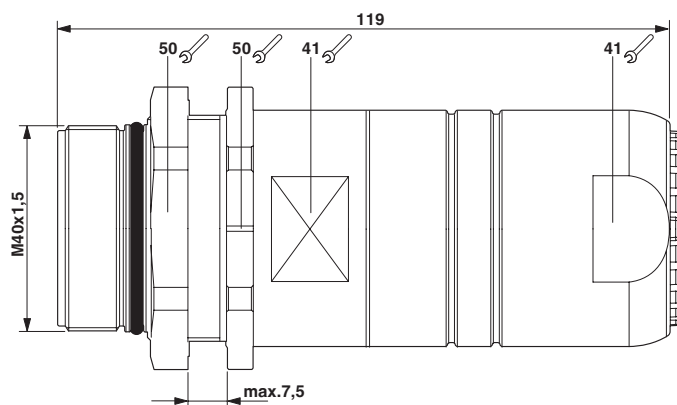
Disegno quotato
