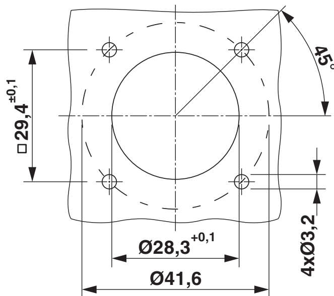
Disegno quotato
