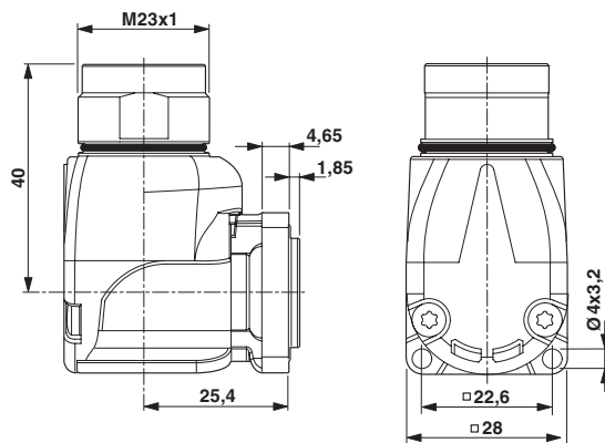
Disegno quotato
