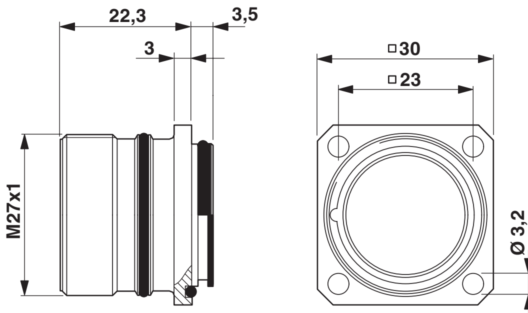
Disegno quotato
