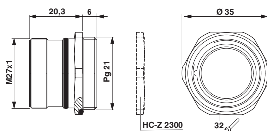
Disegno quotato
