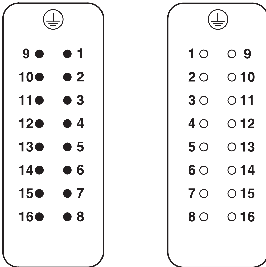
Pinning lato collegamenti
