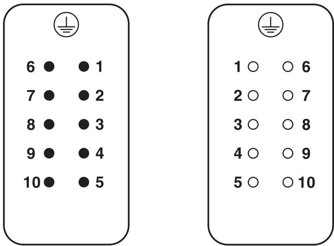
Disegno schema
