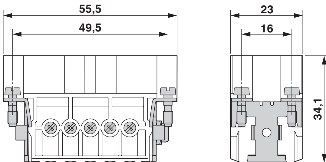
Inserto portacontatti maschio
