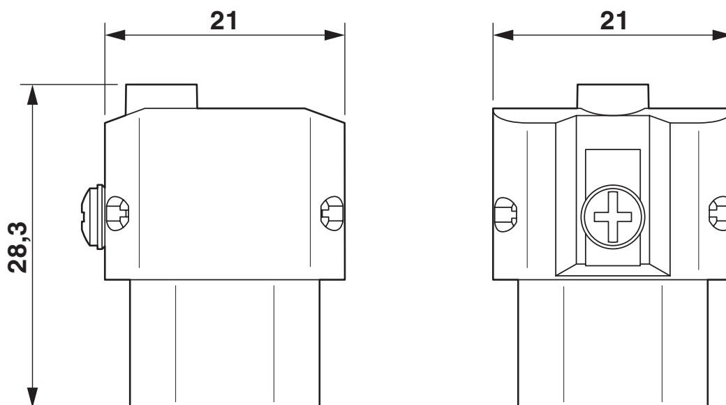
Disegno quotato
