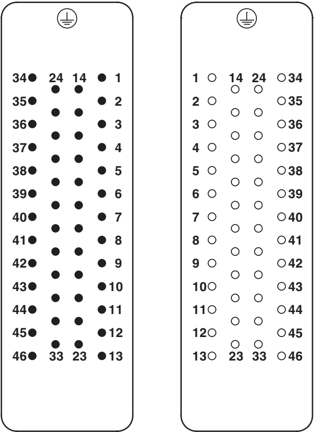
Disegno schema
