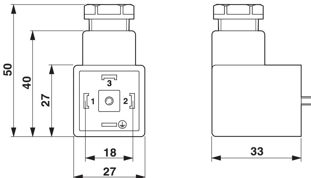
Disegno quotato
