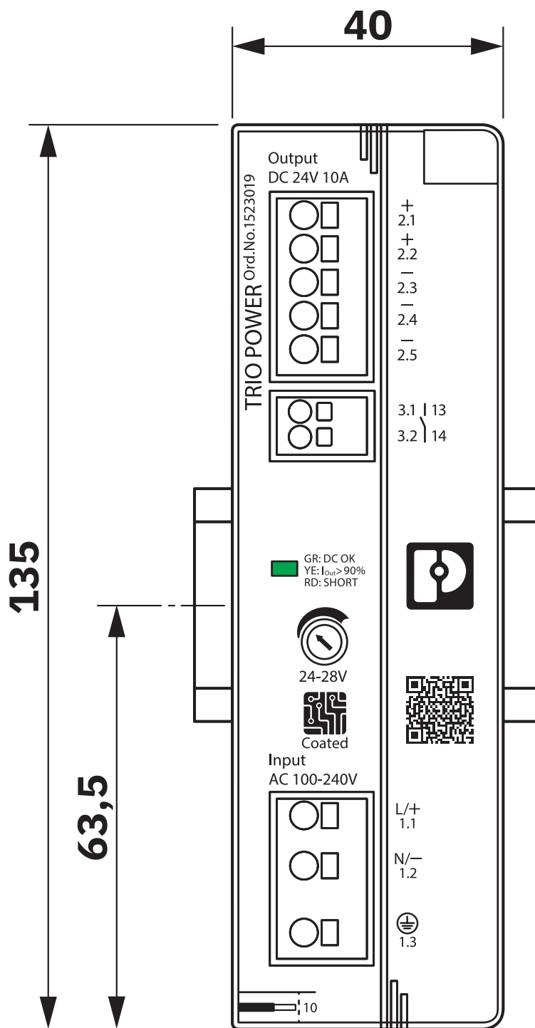
Disegno quotato
