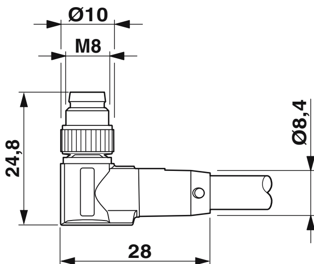
Disegno quotato
