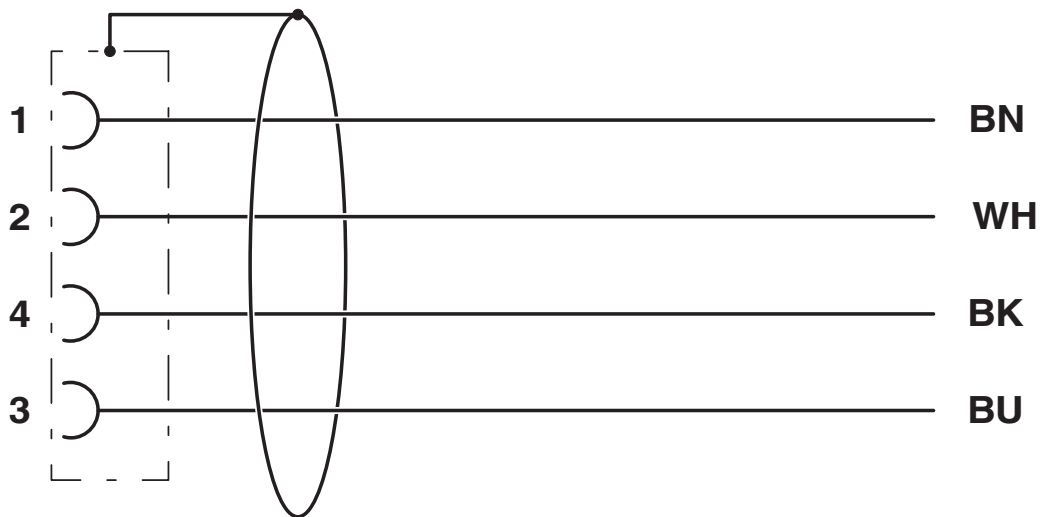
Equipaggiamento dei contatti del connettore femmina M8
