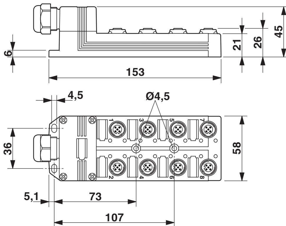
Disegno quotato
