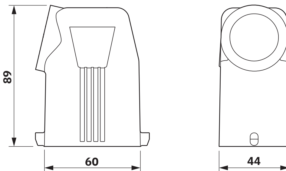
Disegno quotato
