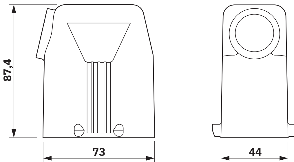
Disegno quotato
