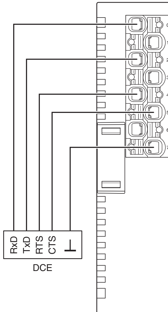
Disegno collegamento
