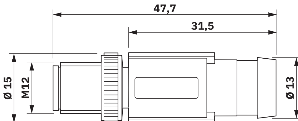
Disegno quotato
