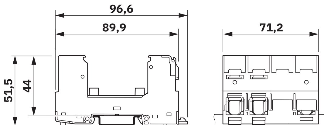
Disegno quotato
