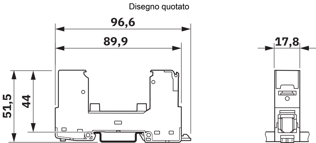
Disegno schema
