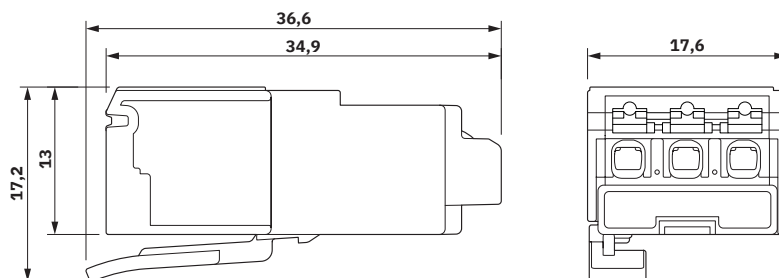
Disegno quotato
