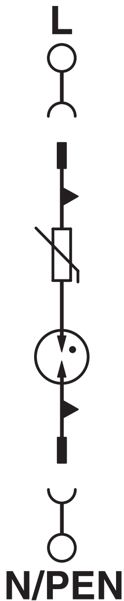
Schema di collegamento
