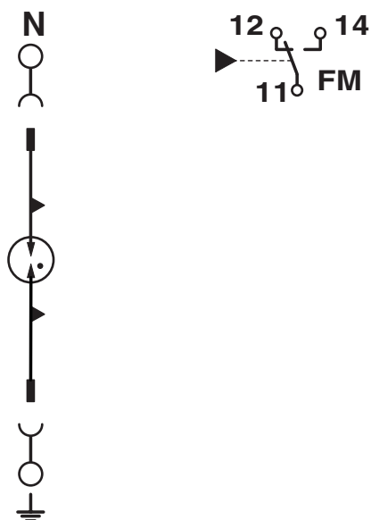
Schema di collegamento
