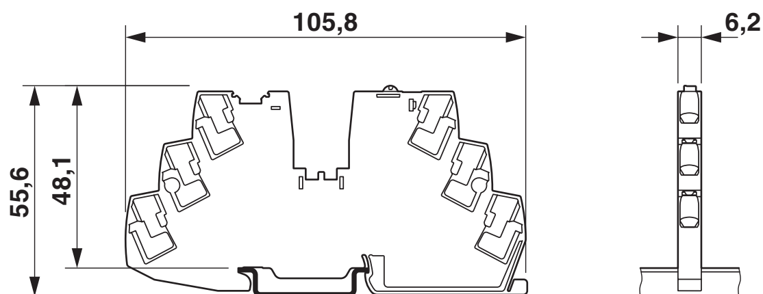
Disegno quotato
