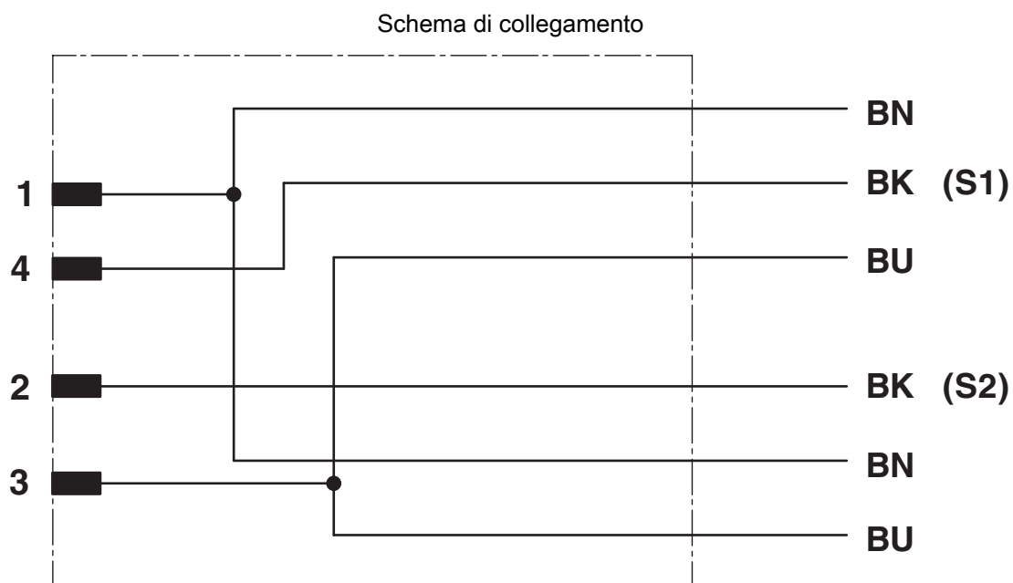
Equipaggiamento dei contatti del distributore M8 a Y
