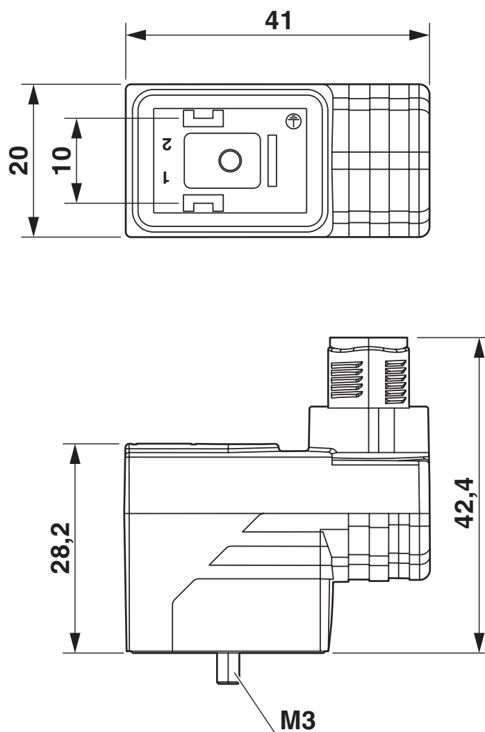
Disegno quotato
