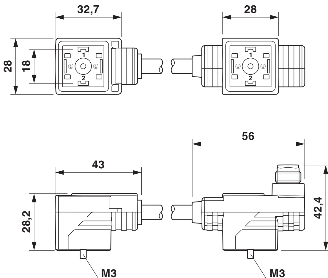
Disegno quotato
