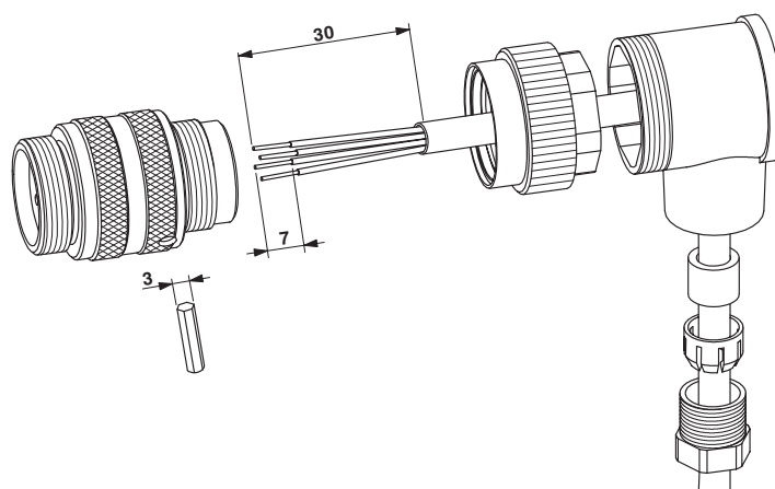
Disegno funzionamento
