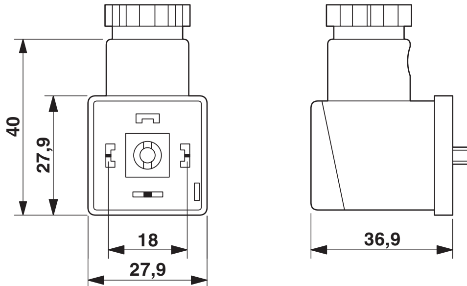
Disegno quotato
