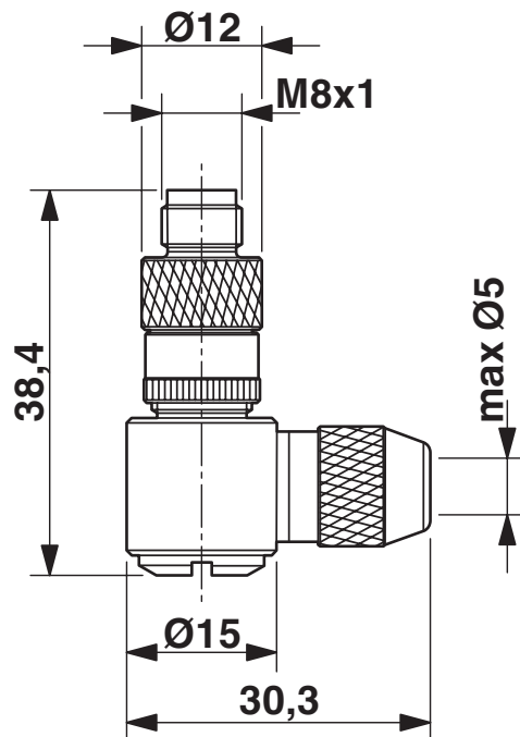
Disegno quotato
