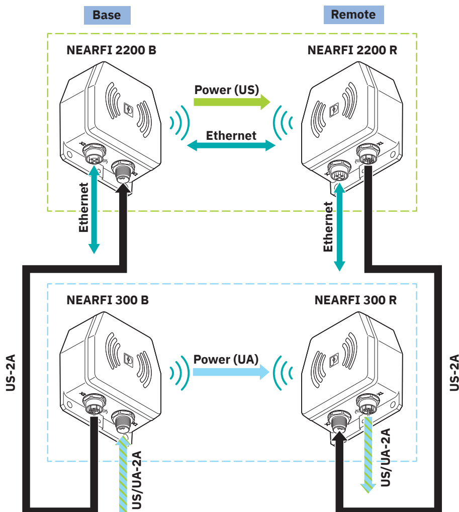
Disegno schema
